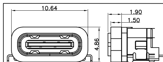
加防水圈示意图
