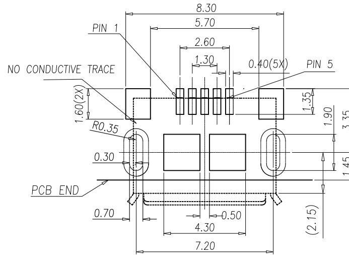
PCB LAYOUT(±0.05)
