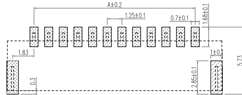
印制线路板
