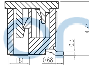
截面 A-A
