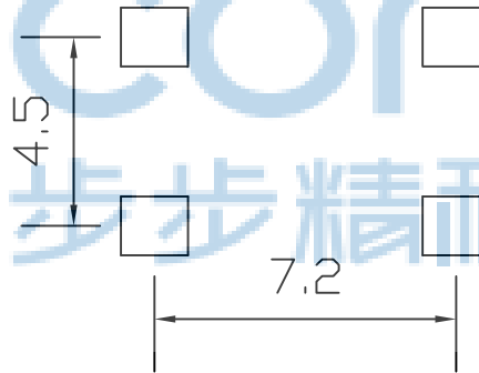
安装尺寸
