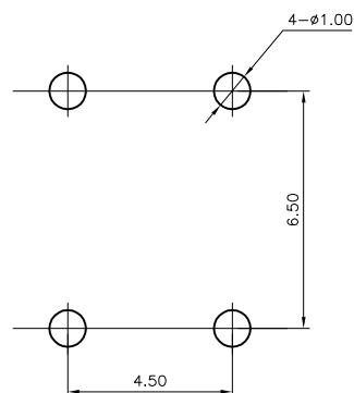
PCB. 焊接图
