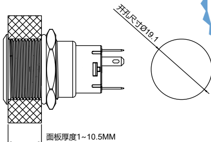
安装视图
