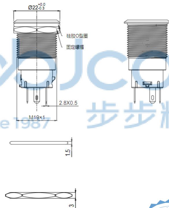
安装视图
