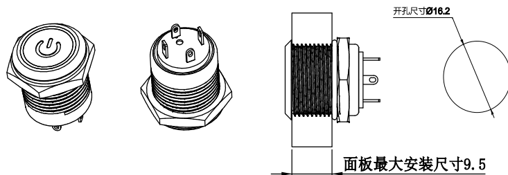
轴视图
