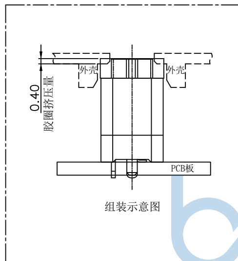
组装示意图
