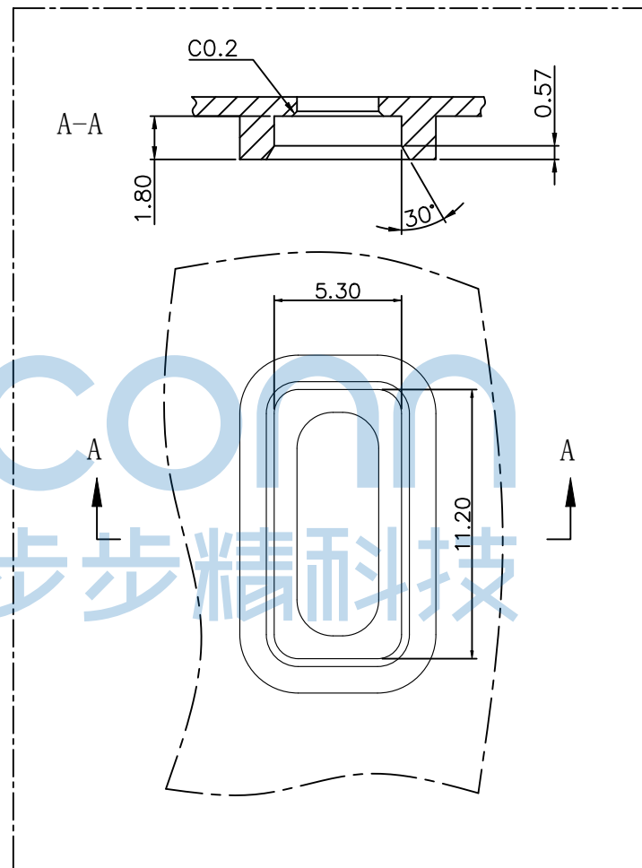
外壳参考设计图
