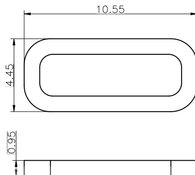
防水圈图示
