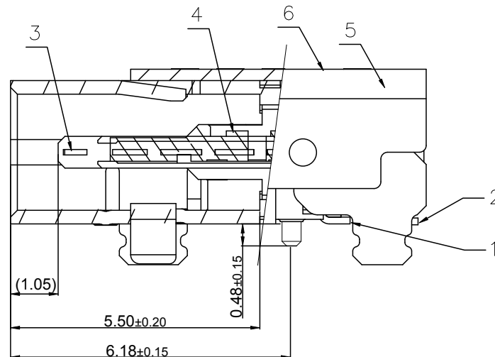
SECTION A-A(剖视图A-A) SCALE 2:1 (比例 2:1)
