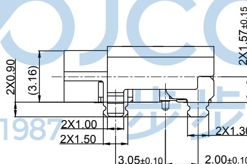
SECTION A-A(剖视图A-A) SCALE 2:1 (比例 2:1)
