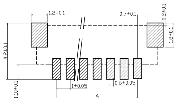
1.0LT-nP PCB寸法 PCB Layout
