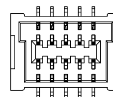
2*5P结构样式
