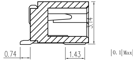
截面 A-A
