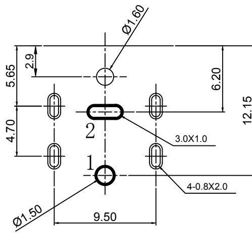
P. C. B 设计参考尺寸
