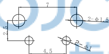
PCB参考图
