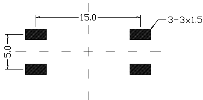
PCB线路板图
