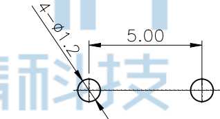
PCB线路板安装图(±0.1)
