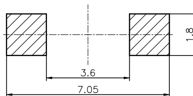
安装参考图
