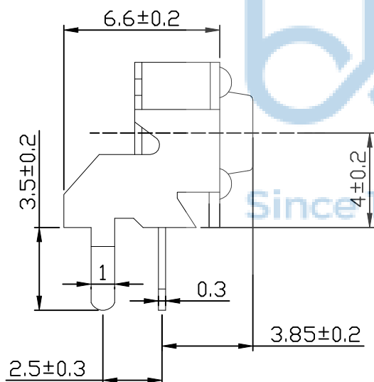
PCB. 安装图
