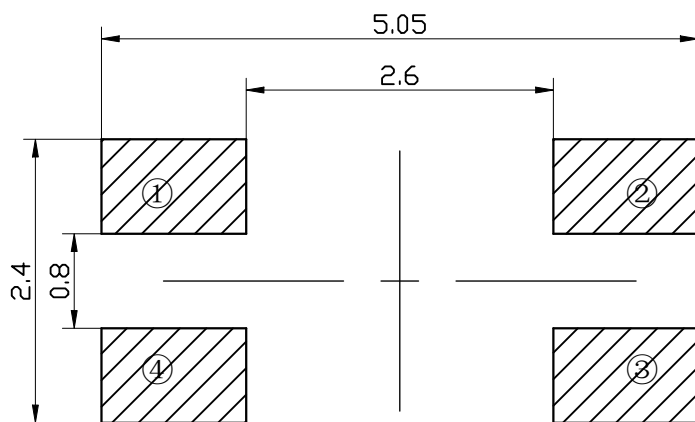
安装参考图
