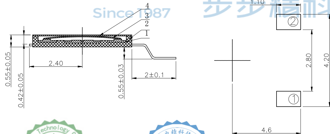
安装参考图
