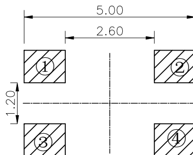
安装参考图
