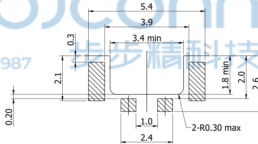
P.C.B LAND DIMENSION
