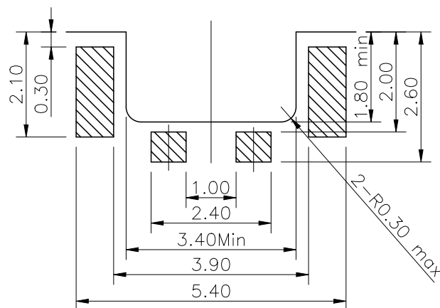
安装参考图
