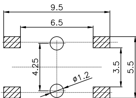
PCB线路板安装图( \pm 0.1 )
