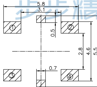
安装参考图
