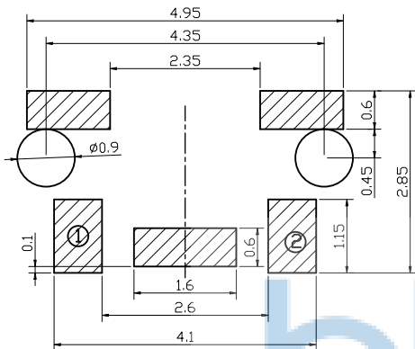
安装参考图
