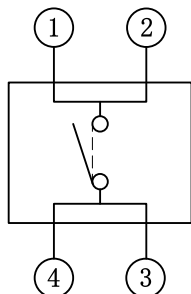
电路图：常开式(N.O) 1个电路1个触点 端子排列（自A方向看）
