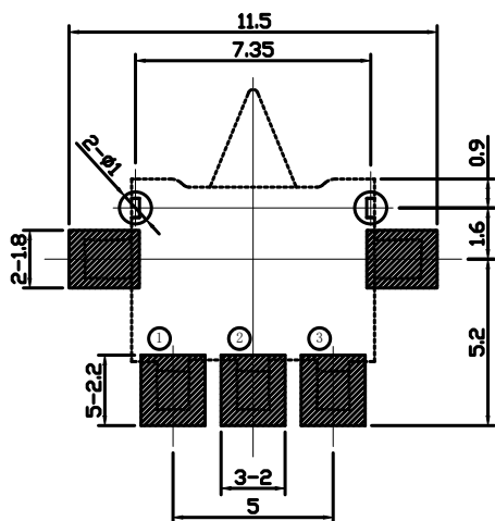
安装尺寸
