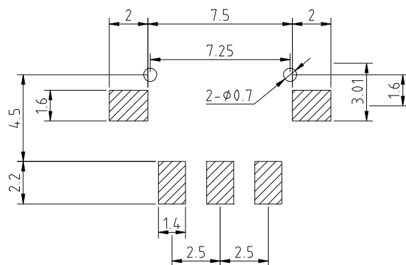
印制电路板及焊接安装孔参考图
