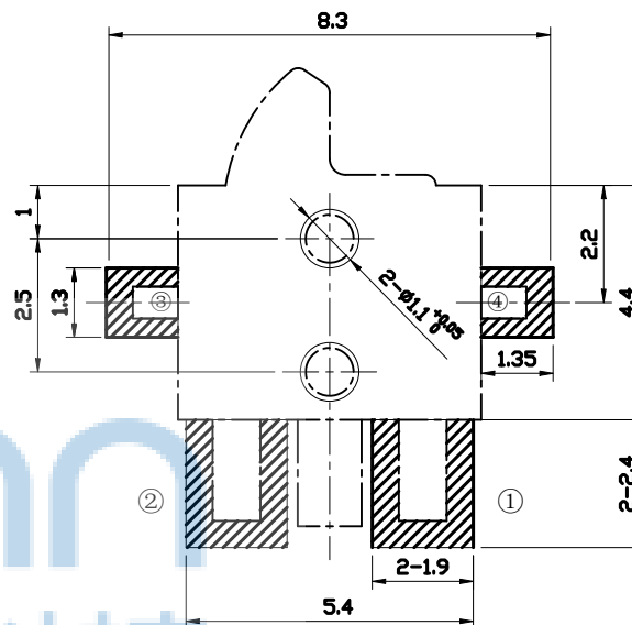
安装位置图
