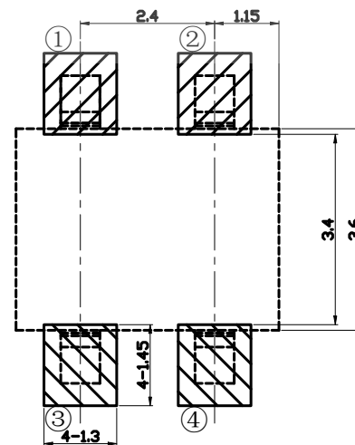
安装位置图
