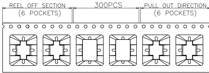
① 产品入载带示意图
