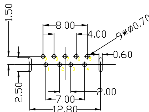
P.C.B LAYOUT TOL:±0.05
