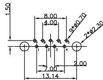
P.C.B LAYOUT TOL:±0.05
