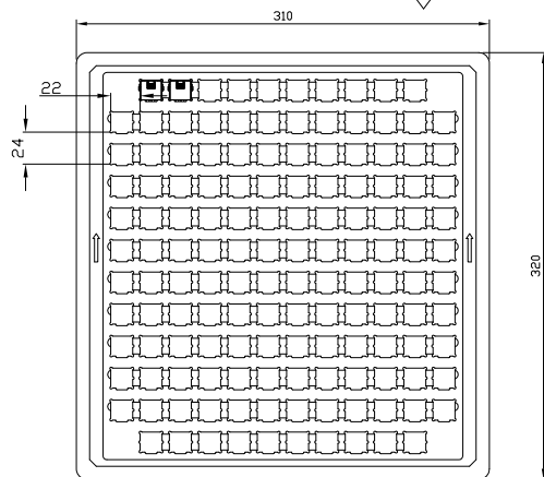
底座
