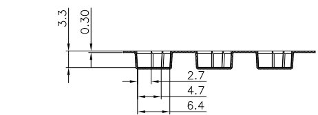
SECTION A-A SCALE 1:1
