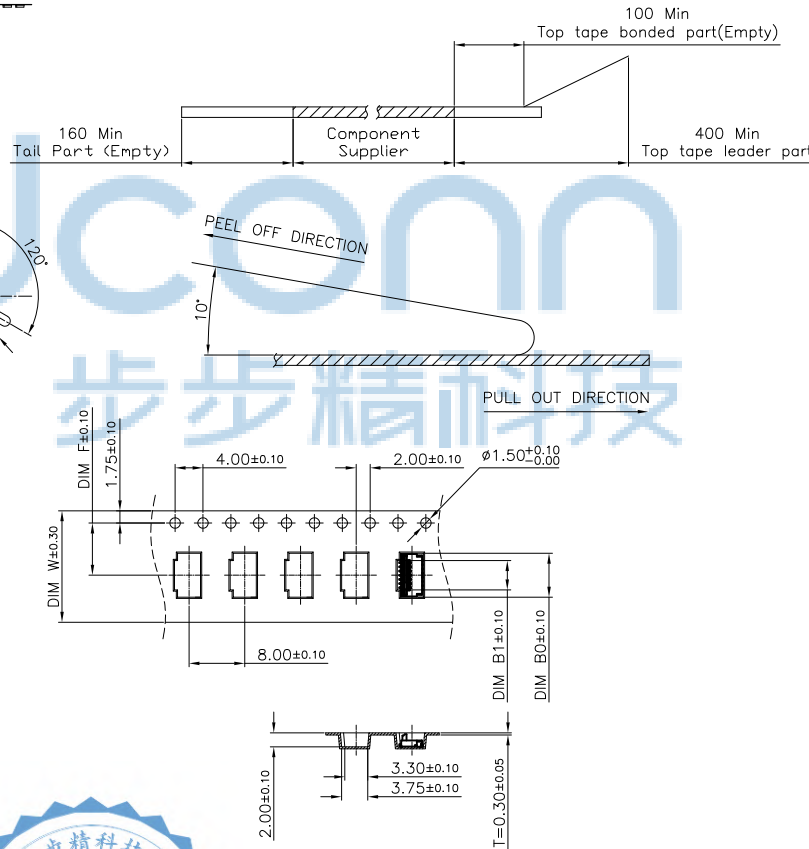
9~47PIN REEL
