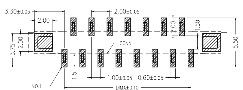
适用线路板 (PCB LAYOUT)
