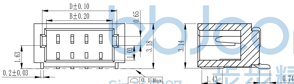
截面 A-A
