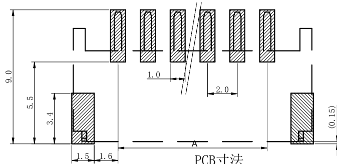
PCB寸法 PCB Layout
