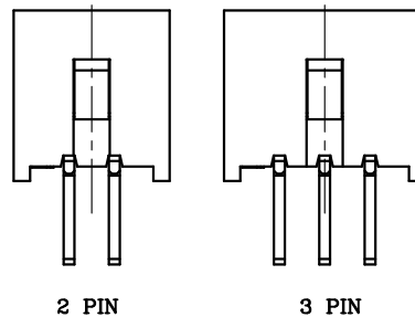
LOCK CONFIGURATION (锁扣位置)
