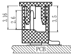
剖面 A-A
