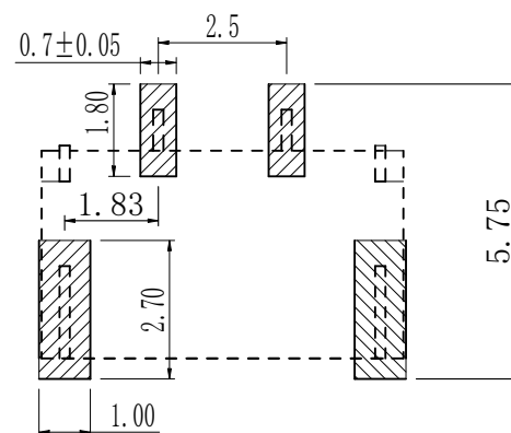
印制线路板
