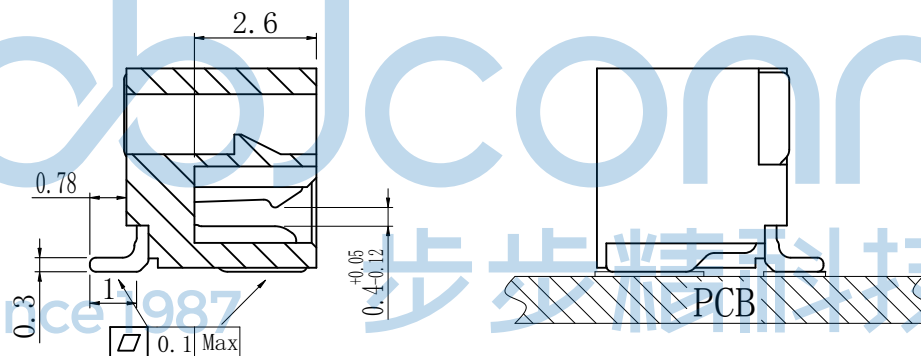
剖面 A-A
