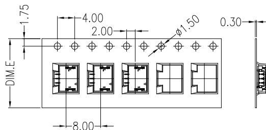
产品引出方向 03~12 CONTACTS
