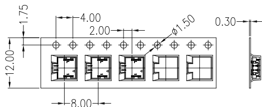
产品引出方向 02 CONTACTS
