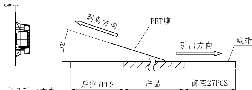
(PET膜剥离示意图)
