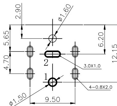
P.C.B 设计参考尺寸
