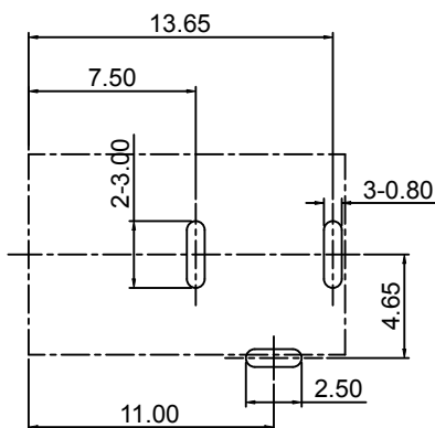
P.C.B 设计参考尺寸
