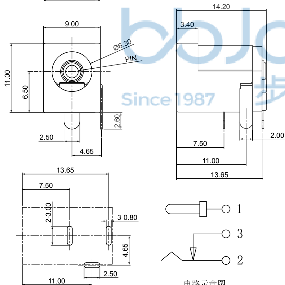
P.C.B 设计参考尺寸
