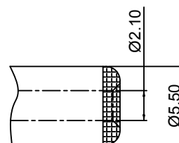
推荐插头尺寸
