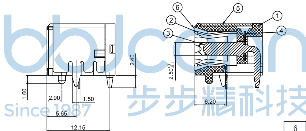
P.C.B 设计参考尺寸
